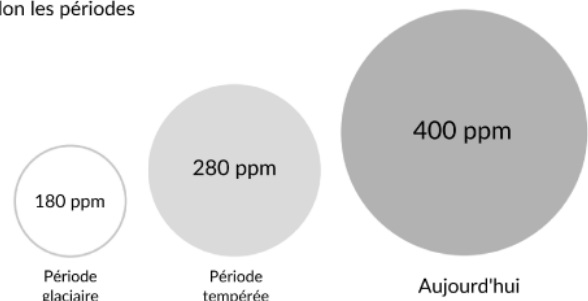
Proportion de dioxyde de carbone dans l'atmosphère selon les périodes
